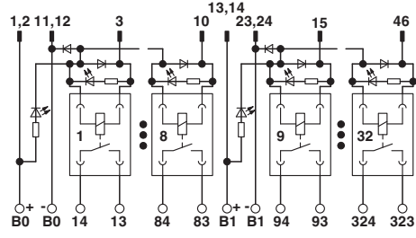
Devre şeması
